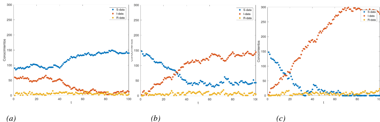
Figura 11: Resultados de la simulación un proceso de enseñanza-aprendizaje según la variante SAOS correspondiente al modelo SIRS.
