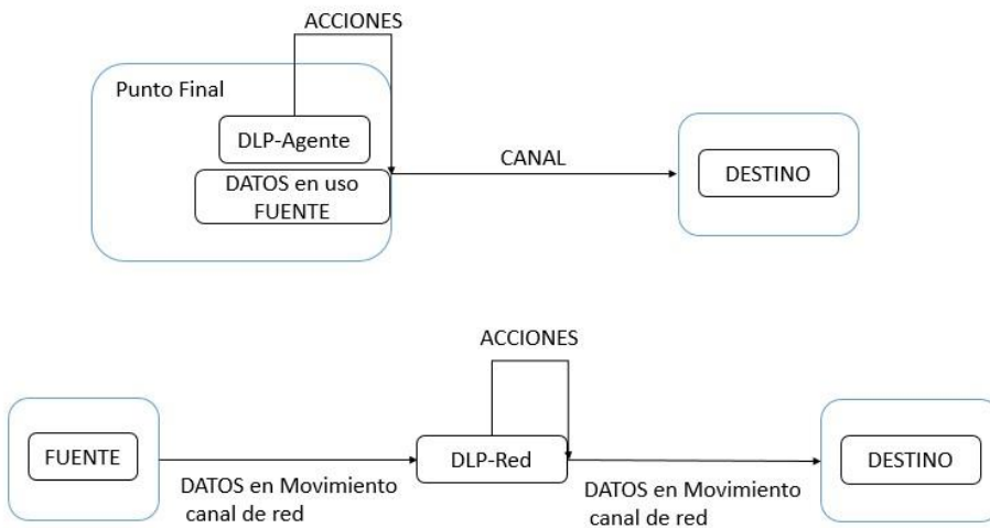
Figura 7: DLP- Punto final para datos en uso y DLP-Red para datos en movimientos. Modelo DLP
